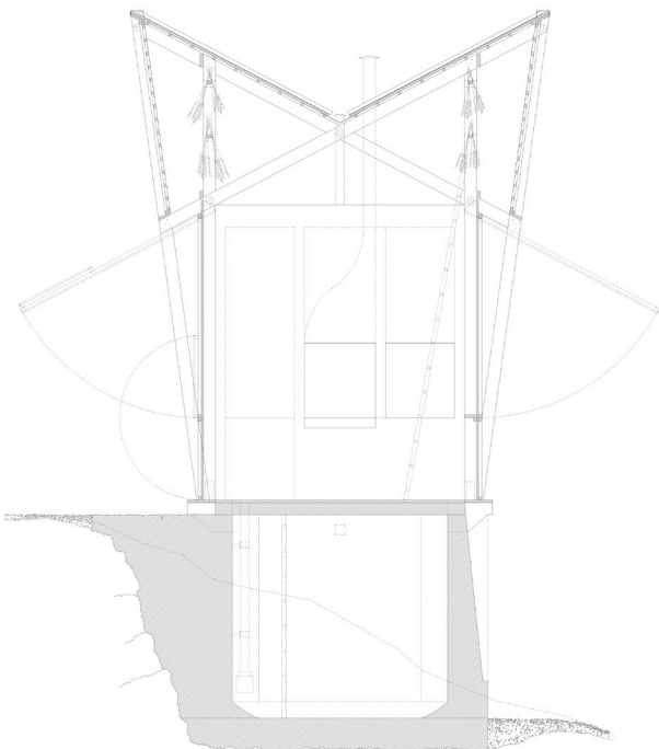
Coupe transversale AA' - échelle 1.50 -
